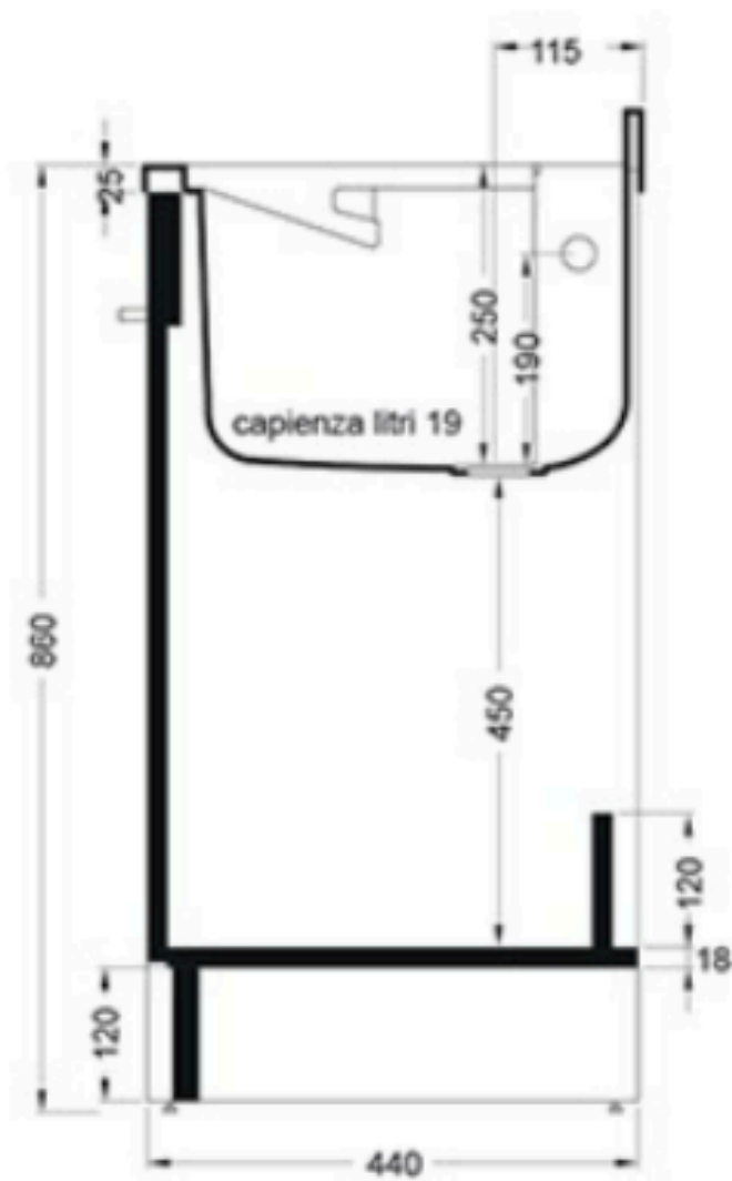
SEZIONE A-A
