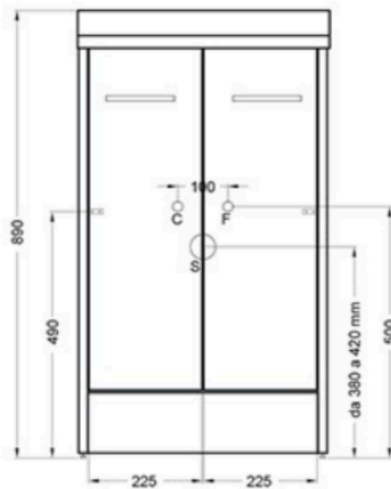
VISTA FRONTALE
