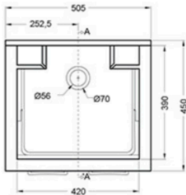
PIANTA
